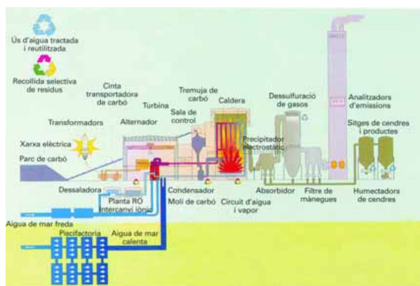
Esquema de la instal·lació .
